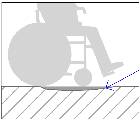
superficie con giunti < a 5 mm risalti < a 1 mm
